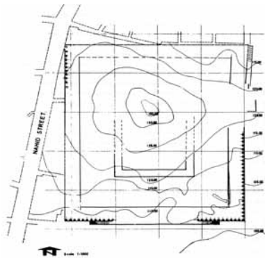
تصویر شماره ۳: وضعیت معماری به دست آمده از معبد آناهیتا پس از کاوش‌ها، ترسیم در دفتر معماری کنگاور توسط محمد مهریار (مأخذ: کامبخش‌فرد، ۱۳۷۴)
